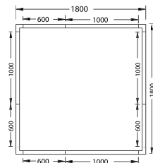
Elementrum C: 180 x 180 cm, CU 450
