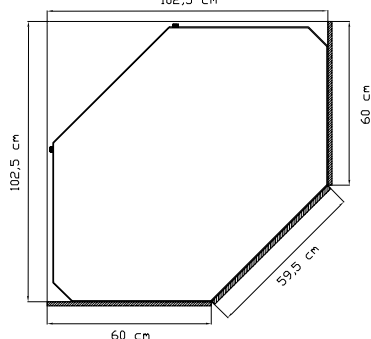
Ritningen visar platsering av hörnkylen brevid skåp med 60cm djup.
