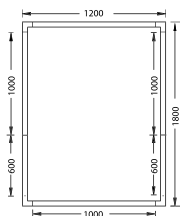
Elementrum B: 120 x 180 cm, CU 350
