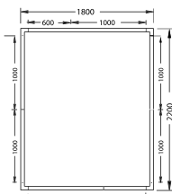
Elementrum D: 180 x 220 cm, CU 450
